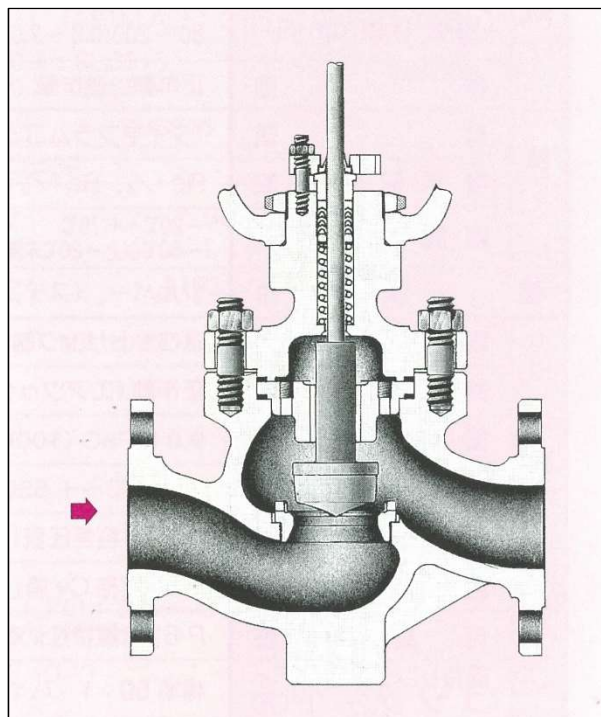
【注】本図は 40A 以上のプレーンボンネット形構造を示します。
